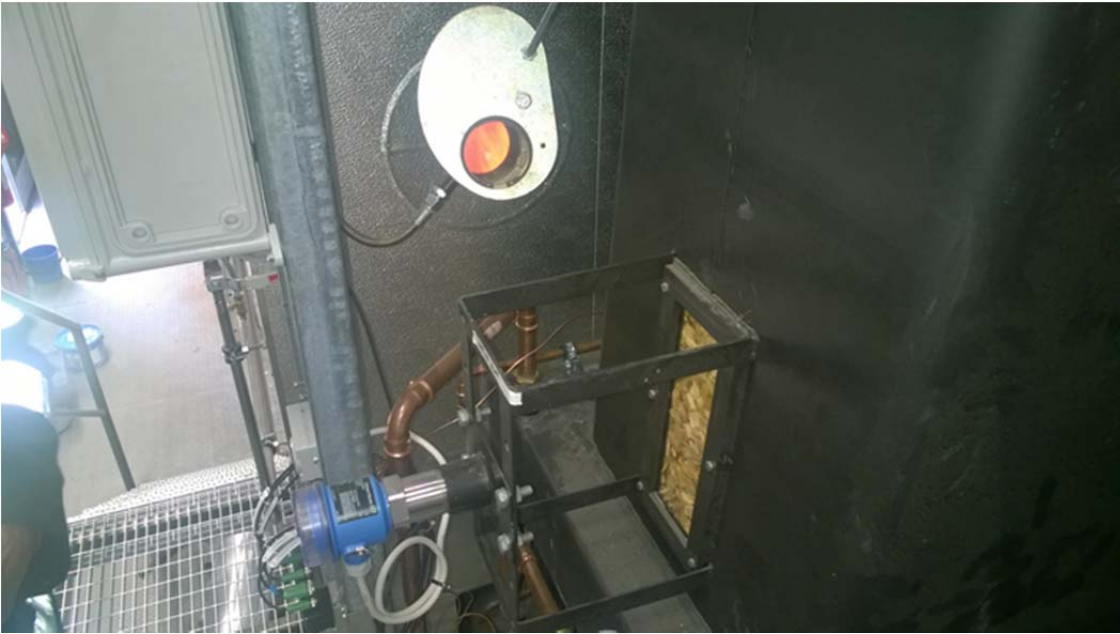
Haketta Immolan kattilan syöttösuppilossa ja palamassa arinalla
